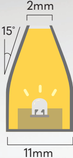
LumiMini - Beveled Edges
